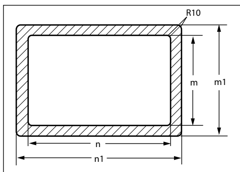
Wymiary wycięcia Kiora, Vero
